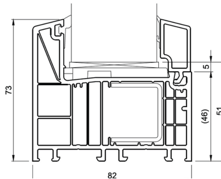
Vlak profiel 82 Doorsnede vast raam Zonder aanslag
