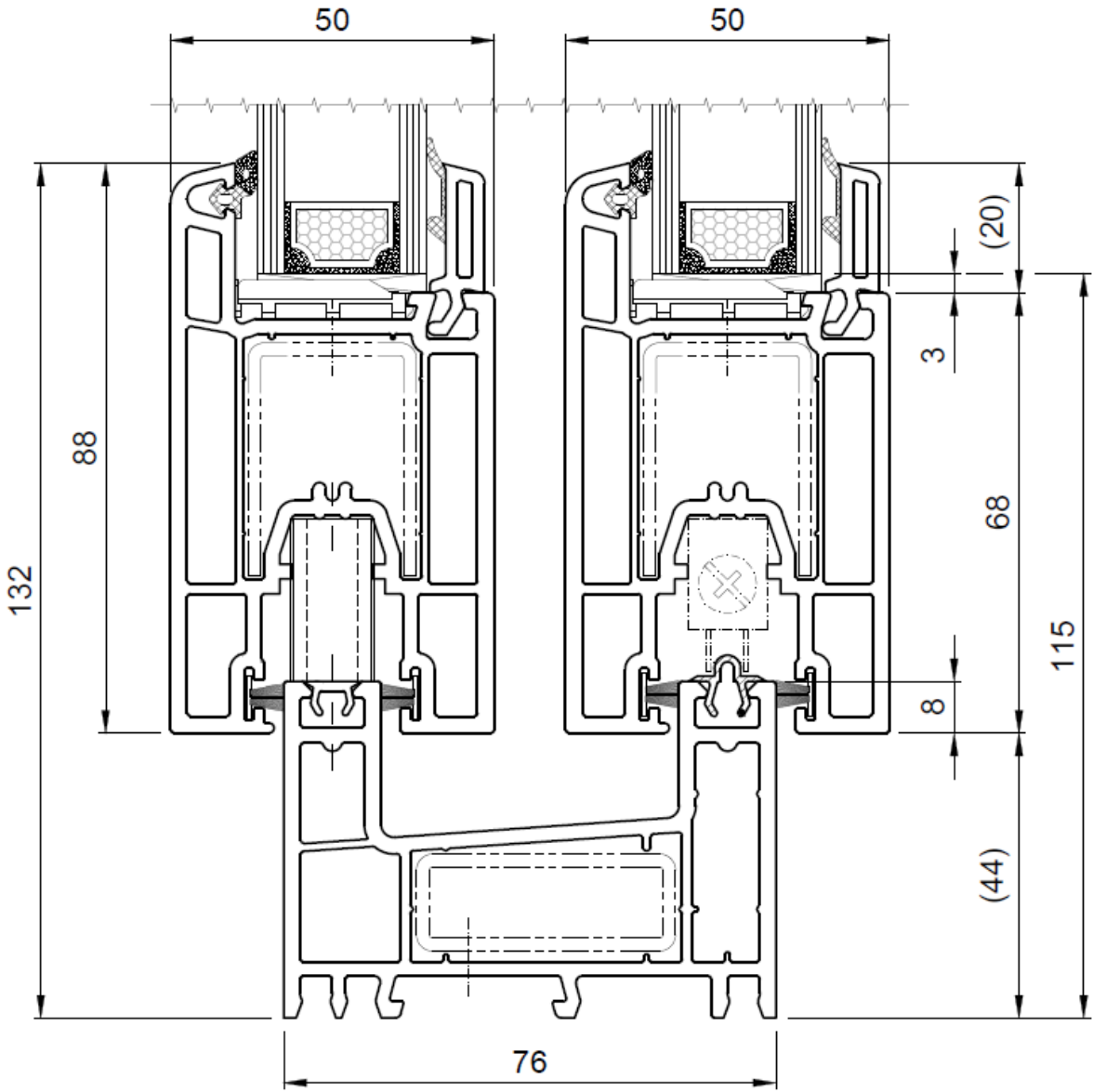
Creon schuifpui zonder aanslag, EvolutionDrive SF, onderdetail
