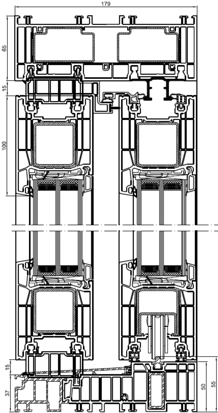
Doorsnede tekening Premidoor 76
